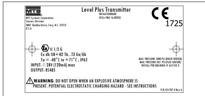
Fig. 58: Druckfest, ATEX- und IECEx-Kennzeichnung, Modbus oder DDA, Gehäuseoption D, E, G, H oder L
