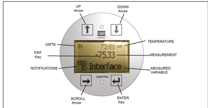
Fig. 6: Display
