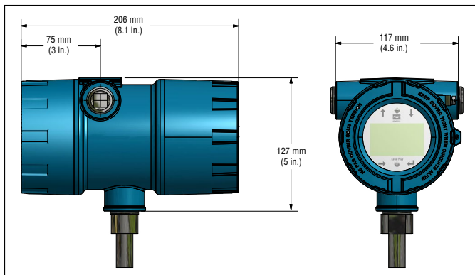
Fig. 2: Duales Hohlraumgehäuse
