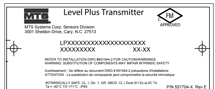
Fig. 33: FMC-Kennzeichnung Eigensicherheit, HART®, einzelnes oder duales Hohlraumgehäuse
