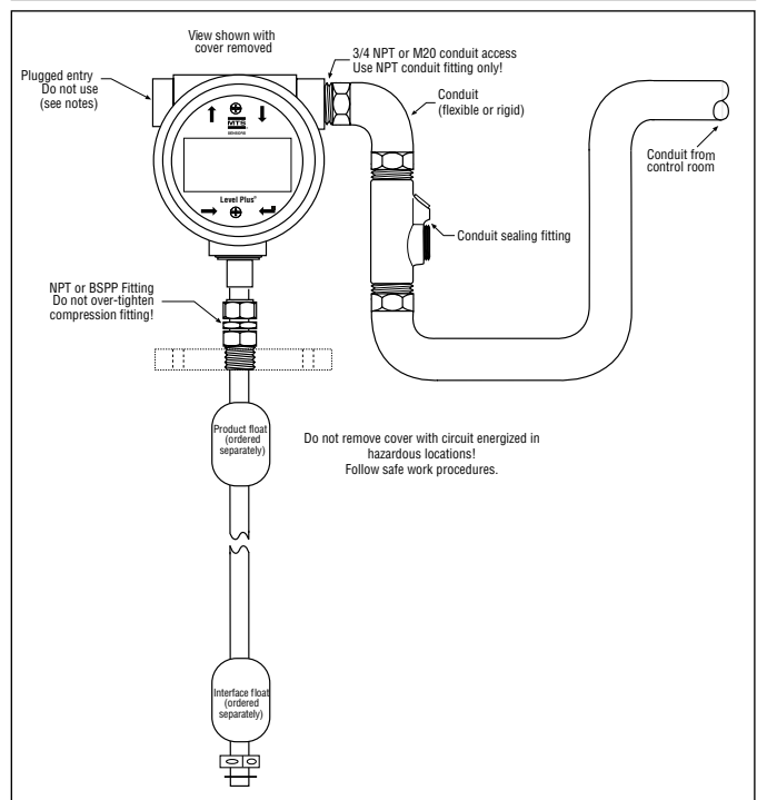
Fig. 13: Installation des Kabelkanals
