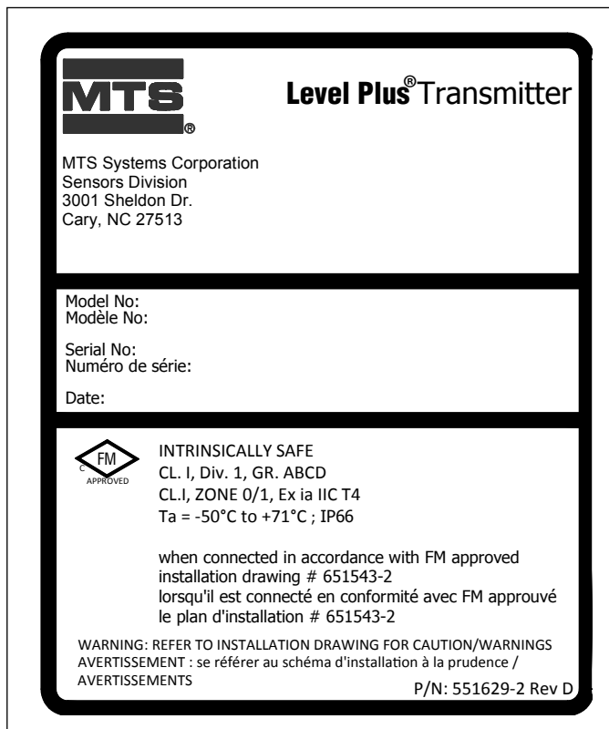
Fig. 30: FMC-Kennzeichnung Eigensicherheit, Modbus und DDA, NEMA-Gehäuse
