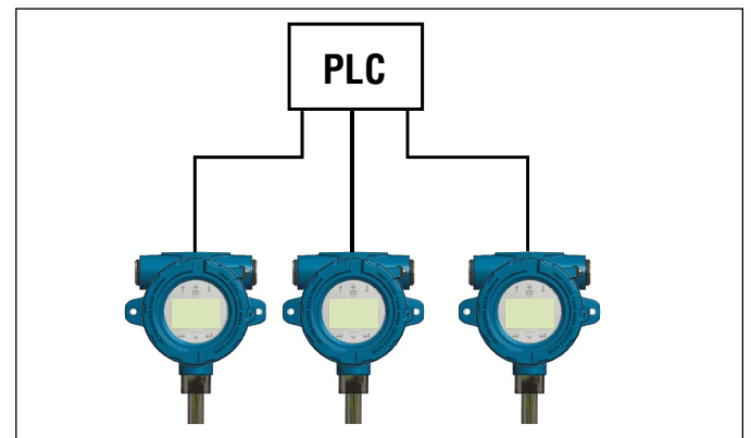
Fig. 8: Punkt-zu-Punkt-Topologie
