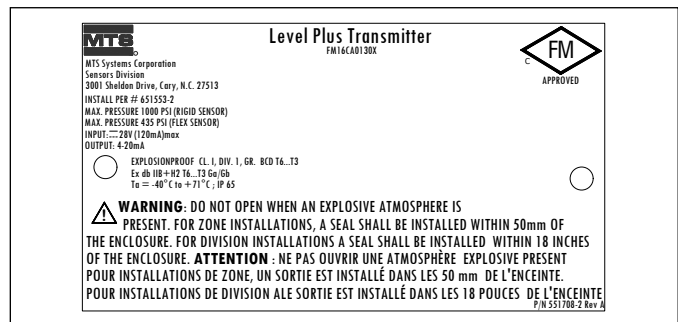
Fig. 43: Explosionsgeschützt, FMC-Kennzeichnung, HART®, Gehäuseoption D, E
