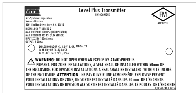
Fig. 42: Explosionsgeschützt, FMC-Kennzeichnung, HART®, Gehäuseoption G, H oder L
