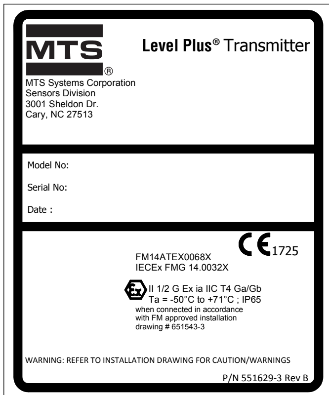
Fig. 50: FMC-Kennzeichnung Eigensicherheit, Modbus und DDA, NEMA-Gehäuse
