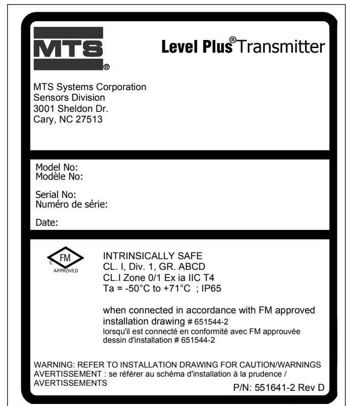
Fig. 31: FMC-Kennzeichnung Eigensicherheit, HART®, NEMA-Gehäuse
