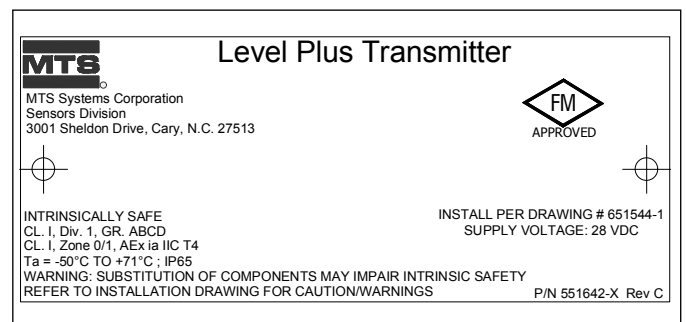
Fig. 17: FM-Kennzeichnung Eigensicherheit, HART®, einfaches oder duales Hohlraumgehäuse
