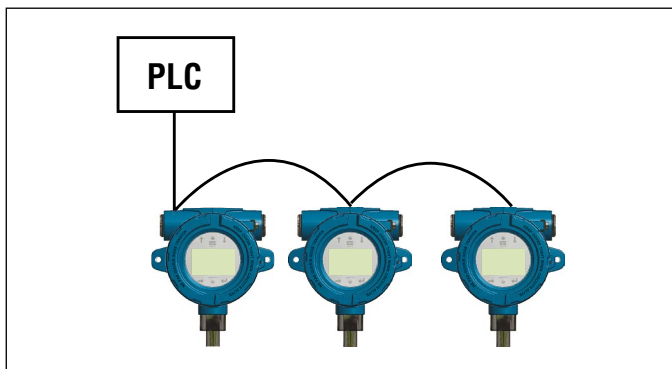
Fig. 12: Daisy-Chain-Topologie
