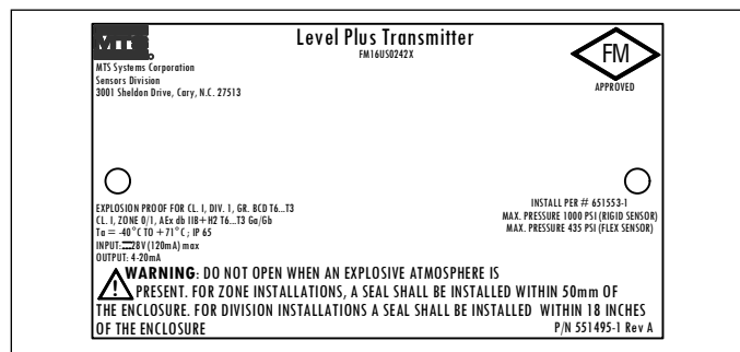
Fig. 24: Explosionsgeschützt, FM-Kennzeichnung, HART®, Gehäuseoption G, H oder L
