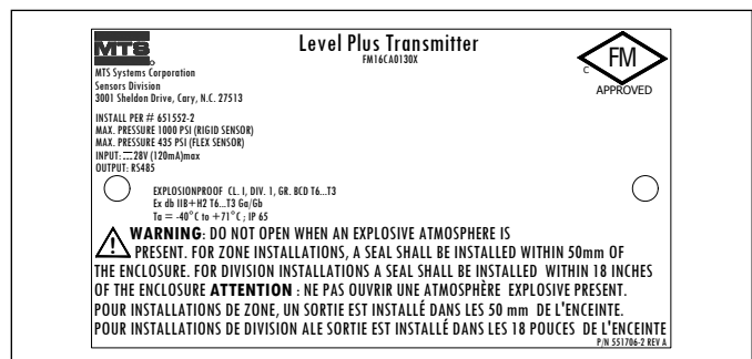
Fig. 41: Explosionsgeschützt, FMC-Kennzeichnung, Modbus oder DDA, Gehäuseoption D, E
