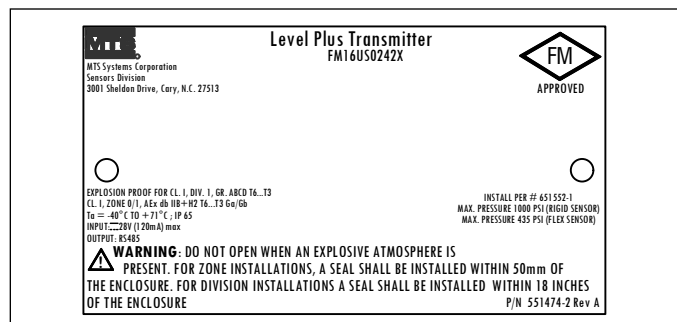
Fig. 23: Explosionsgeschützt, FM-Kennzeichnung, Modbus oder DDA, Gehäuseoption D, E
