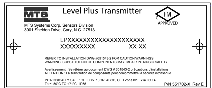
Fig. 32: FMC-Kennzeichnung Eigensicherheit, Modbus und DDA, einzelnes oder duales Hohlraumgehäuse
