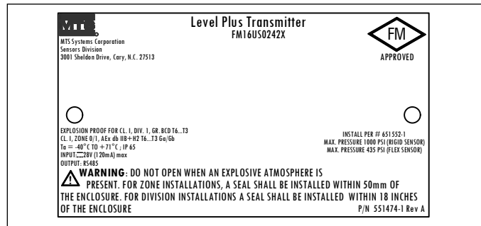
Fig. 22: Explosionsgeschützt, FM-Kennzeichnung, Modbus oder DDA, Gehäuseoption G, H oder L
