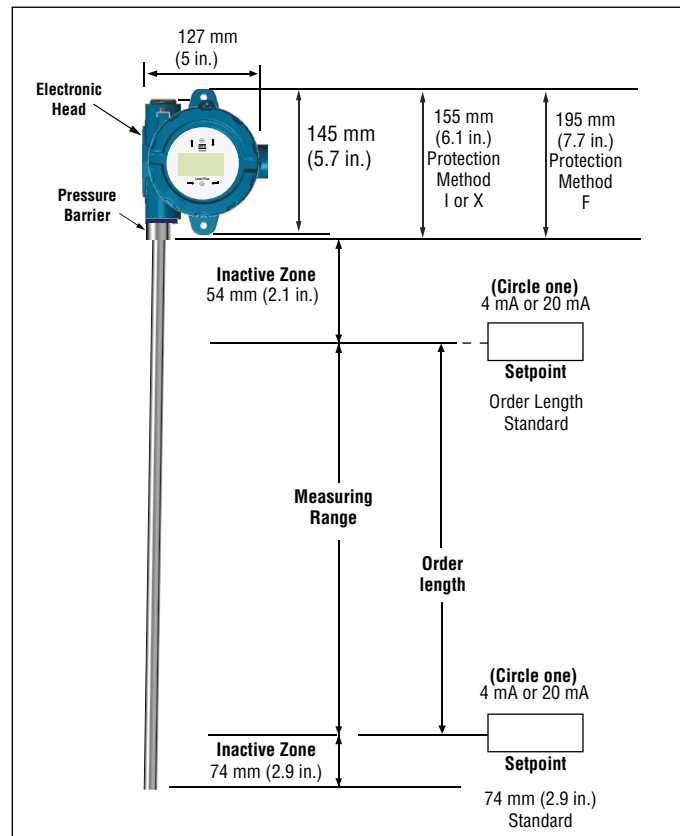
Fig. 7: Montage des CHAMBERED, Bodenflansch
