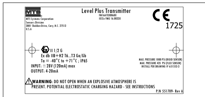
Fig. 59: Druckfest, ATEX- und IECEx-Kennzeichnung, HART®, Gehäuseoption D, E, G, H oder L
