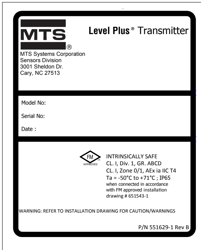
Fig. 14: FM-Kennzeichnung Eigensicherheit, Modbus oder DDA, NEMA-Gehäuse
