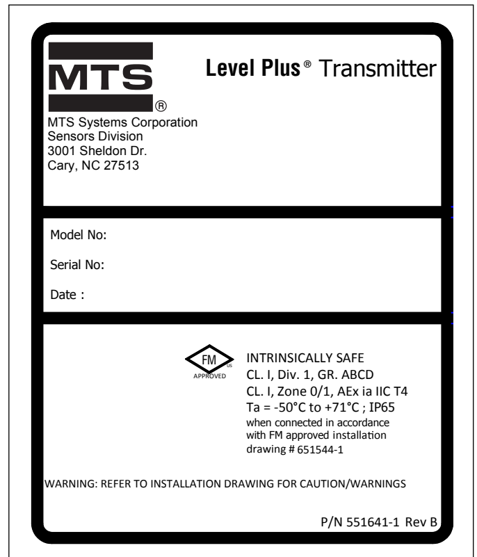
Fig. 15: FM-Kennzeichnung Eigensicherheit, HART®, NEMA-Gehäuse
