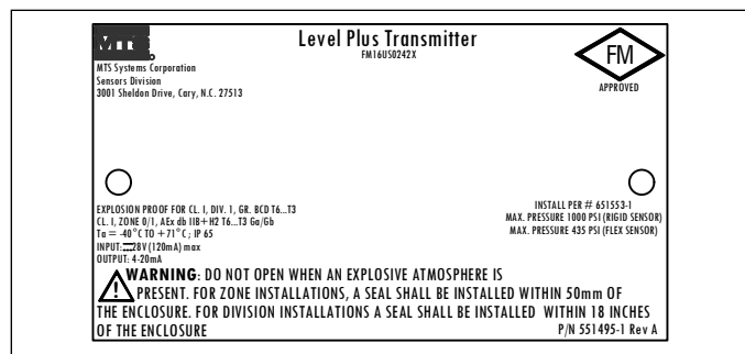
Fig. 25: Explosionsgeschützt, FM-Kennzeichnung, HART®, Gehäuseoption D, E
