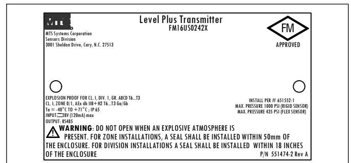
Fig. 24: Antideflagrante, etichetta FM, Modbus o DDA, custodia opzione D, E
