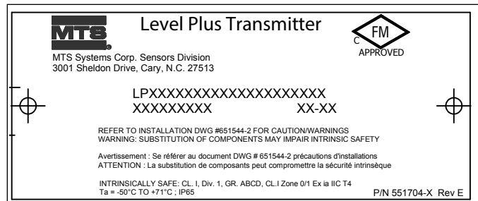
Fig. 34: Etichetta di Sicurezza intrinseca FMC, HART®, custodia con intercapedine singola e doppia
