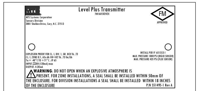
Fig. 25: Antideflagrante, etichetta FM, HART®, custodia opzione G, H o L
