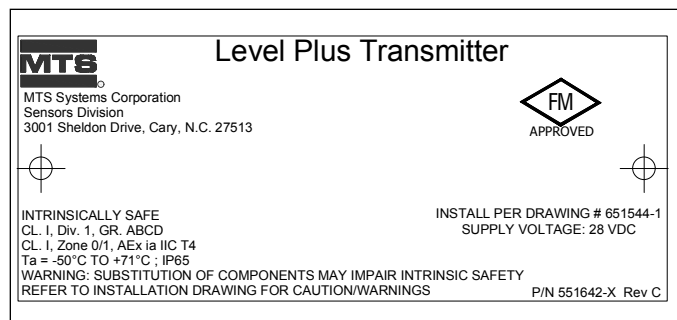
Fig. 18: Etichetta di Sicurezza intrinseca FM, HART®, custodia con intercapedine singola o doppia
