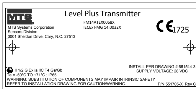
Fig. 54: Etichetta di Sicurezza intrinseca ATEX/IECEx, Modbus e DDA, custodia con intercapedine singola e doppia
