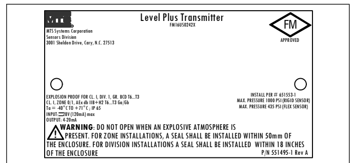
Fig. 26: Antideflagrante, etichetta FM, HART®, custodia opzione D, E
