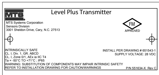
Fig. 17: Etichetta di Sicurezza intrinseca FM, Modbus o DDA, custodia con intercapedine singola o doppia
