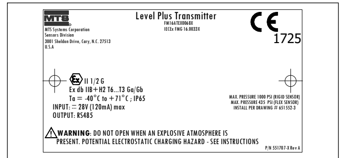
Fig. 59: Ignifugo, etichetta ATEX e IECEx, Modbus o DDA, custodia opzione D, E, G, H o L
