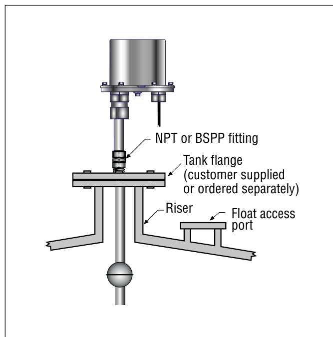
Fig. 8: Montaggio con flangia filettata per tubo flessibile
