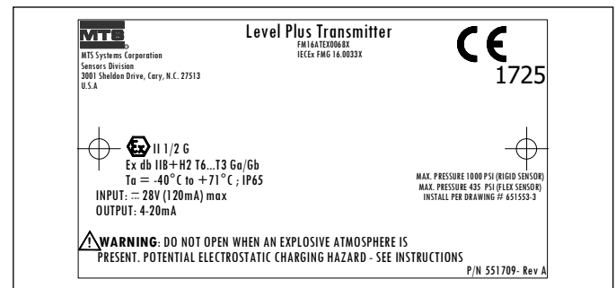
Fig. 60: Ignifugo, etichetta ATEX e IECEx, HART®, custodia opzione D, E, G, H o L
