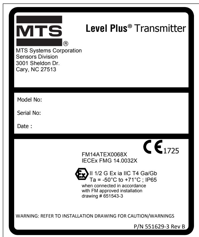
Fig. 51: Etichetta di Sicurezza intrinseca FMC, Modbus e DDA, custodia NEMA
