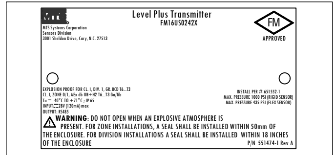
Fig. 23: Antideflagrante, etichetta FM, Modbus o DDA, custodia opzione G, H o L
