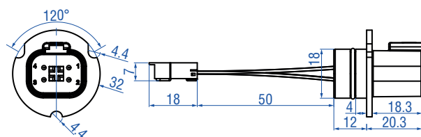
DT-Stecker Artikelnr. 255 098
