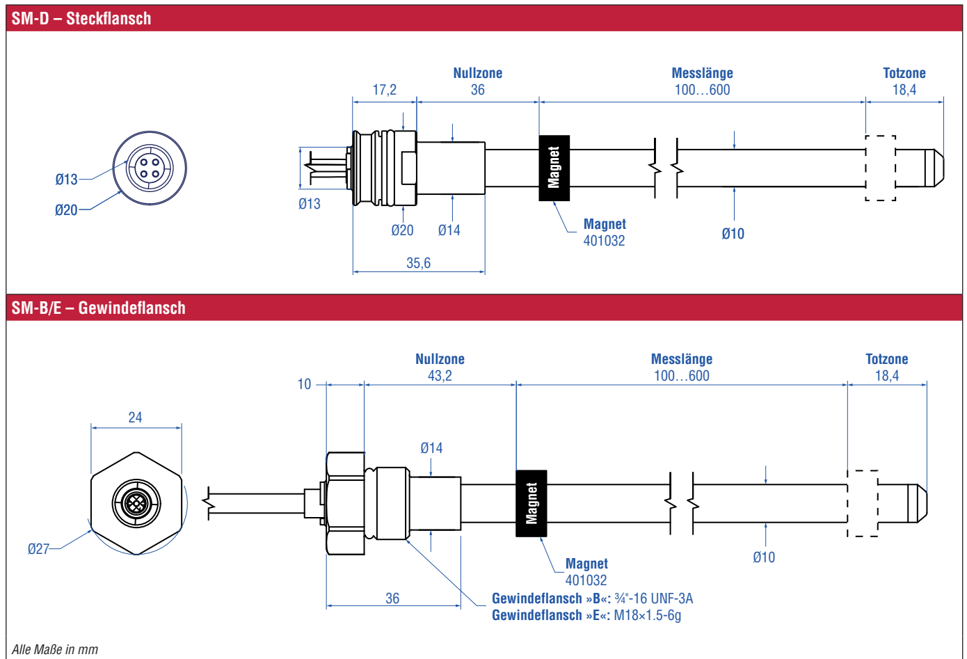
Fig. 3: Temposonics® MH-Serie SLIM Sensor
