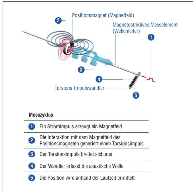
Fig. 1: Laufzeit-basiertes magnetostruktives Positionsmessprinzip
