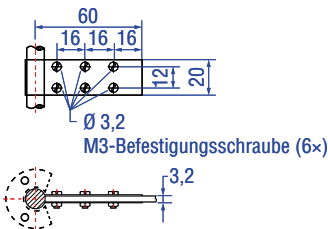
Befestigungslasche Artikelnr. 561 481
