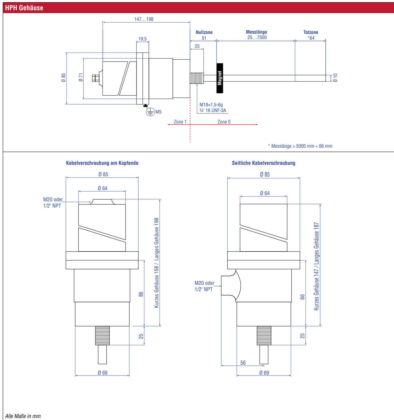
Abb. 4: HPH Gehäuse
