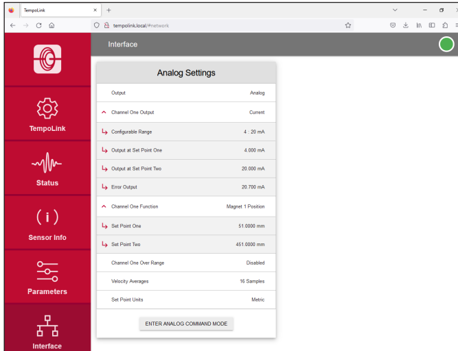
Fig. 84: R-Series V Analog settings
