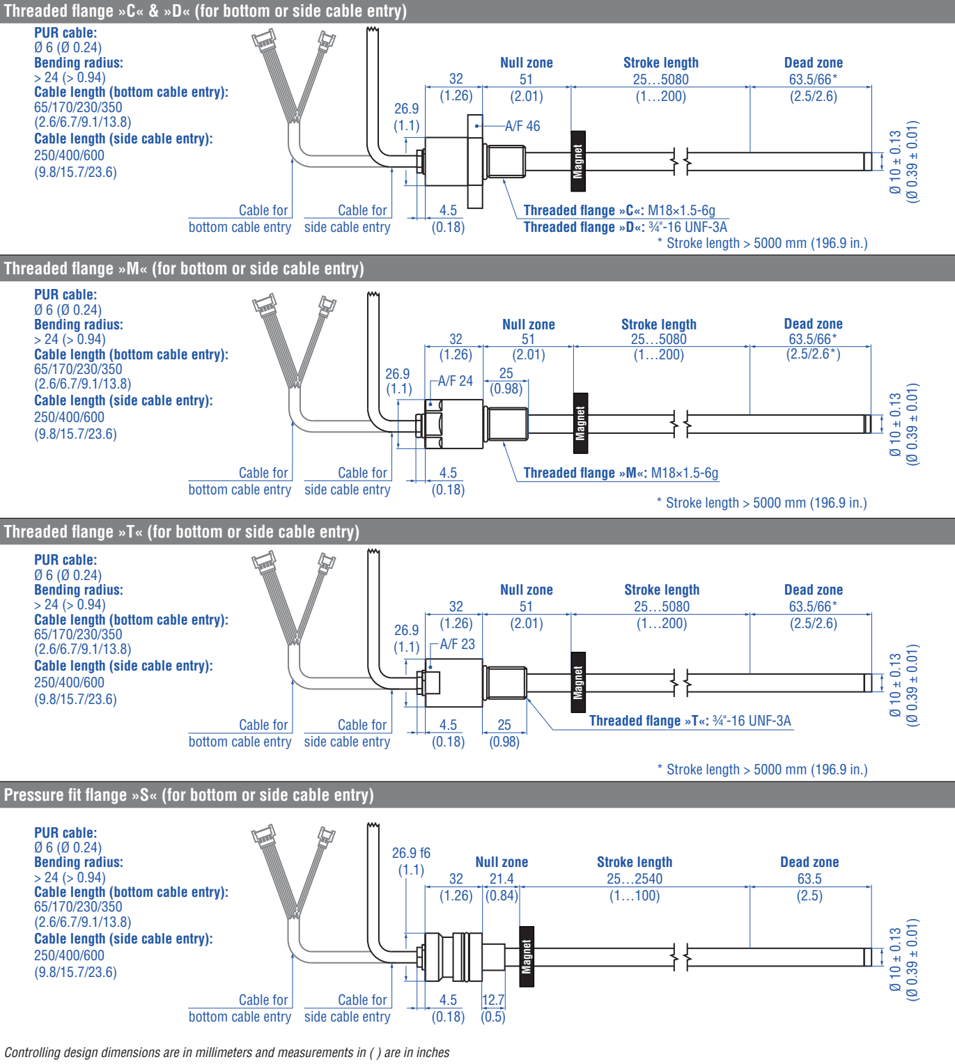
Fig. 27: Temposonics® RDV flanges
